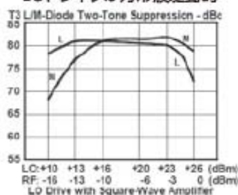
LOドライブが方形波駆動時
