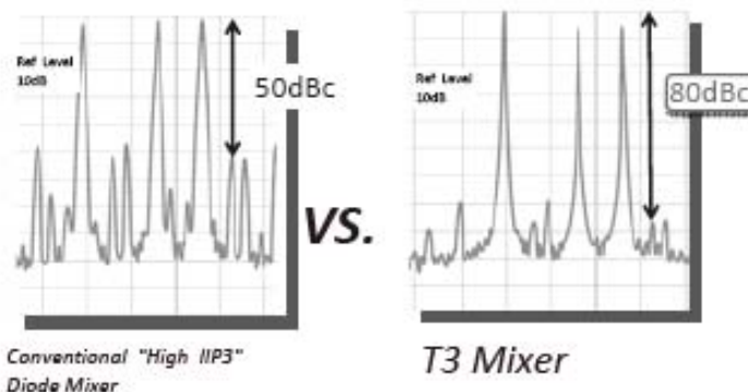
LOドライブがサイン波駆動時
