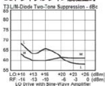
LOドライブがサイン波駆動時
